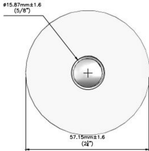
VISTA POSTERIOR escala 1:1
