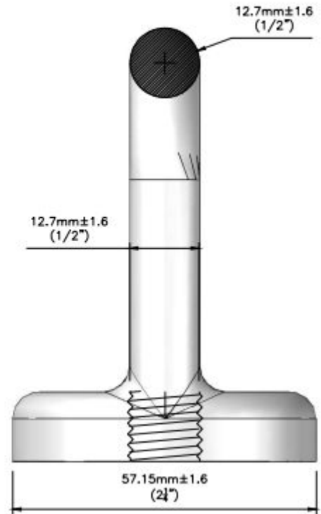
VISTA LATERAL escala 1:1
