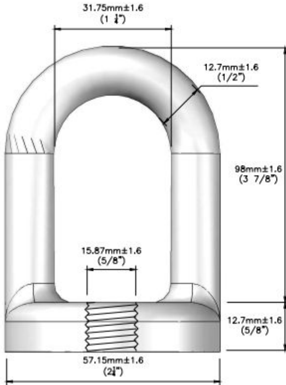
VISTA FRONTAL escala 1:1
